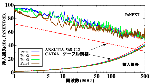
ケーブル特性例 (PsNEXT、挿入損失)
