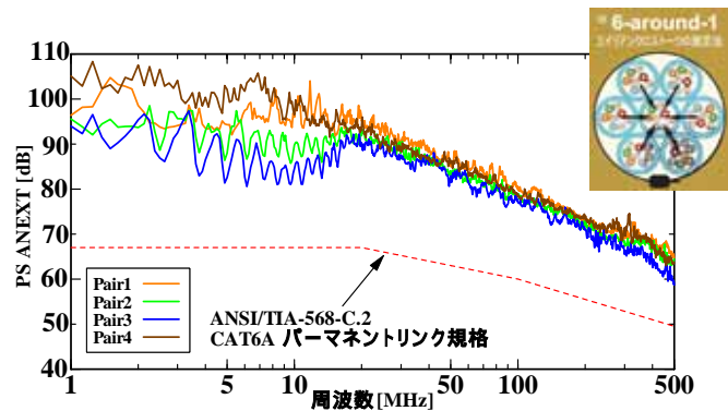
エイリアンクロストーク特性例 (パーマネントリンク90m)
