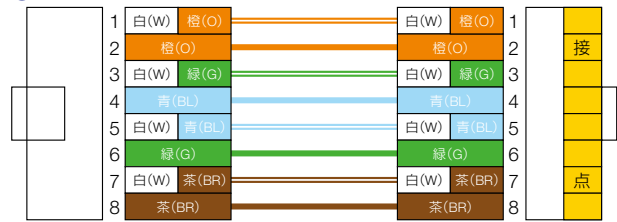
② T568Bストレート
