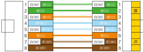
① T568Aストレート
