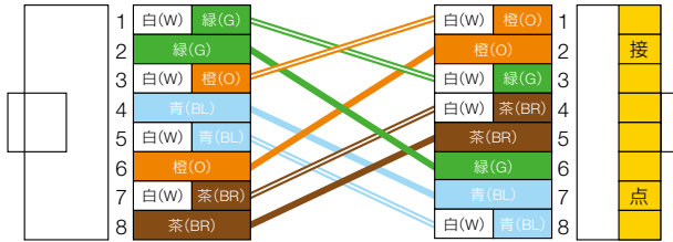
③ 1000BASE-T用 クロスオーバー結線 (IEEE802.3abシステムで使用する結線) T568Aに対してクロスオーバー結線の関係
