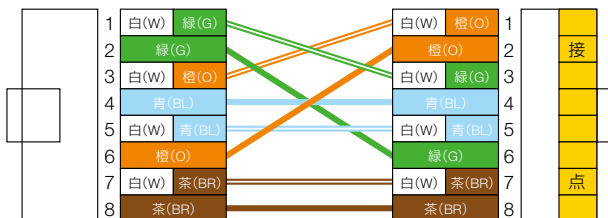
⑦ T568A-Bクロス
