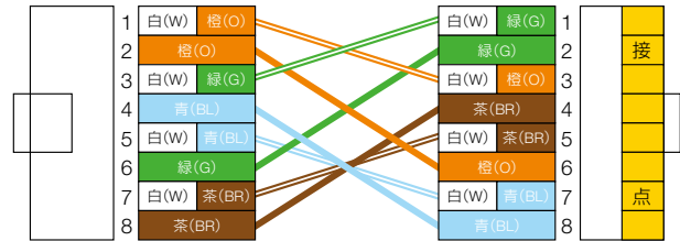
⑥ 1000BASE-TX用 クロスオーバー結線 (TIA/EIA-854のシステムで使用する結線) T568Bに対してクロスオーバー結線の関係
