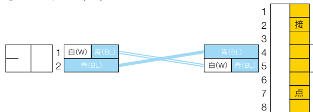
⑨ 110コネクタ(1P)-RJ45
