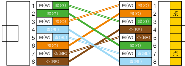
⑤ 1000BASE-TX用 クロスオーバー結線 (TIA/EIA-854のシステムで使用する結線) T568Aに対してクロスオーバー結線の関係
