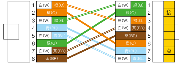
④ 1000BASE-T用 クロスオーバー結線 (IEEE802.3abシステムで使用する結線) T568Bに対してクロスオーバー結線の関係
