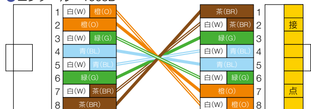
⑧ コンソール T568B
